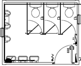
AVTB-1210-01 12' x 10' 3.65m x 3.05m
